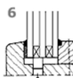
6 Verglasung von Holzfenstern ohne Vorlegeband. Nach der „Richtlinie zur Verglasung von Holzfenstern ohne Vorlegeband, Ziff. 2.1“ aus 9/83 vom Institut für Fenstertechnik, Rosenheim, kann das innere Vorlegeband entfallen, wenn eine entsprechende Nut an der Glasleiste für die innere Versiegelung vorgesehen wird und der Abstand von mindestens 0,5 mm zur Glasdicke eingehalten ist.
