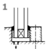
1 Elastische Versiegelung witterungs- und raumseitig auf geschlossenenporigen Vorlegebändern.
