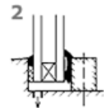
2 Geschlossenenporiges Vorlegeband mit elastischer Versiegelung witterungsseitig und raumseitig in ein Dichtprofil eingerollt oder eingeschoben.
