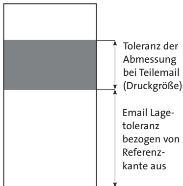
Abb. 19 zu Tab. 21: Fehlerarten/Toleranzen für vollflächig bzw. teilflächig emaillierte Gläser
